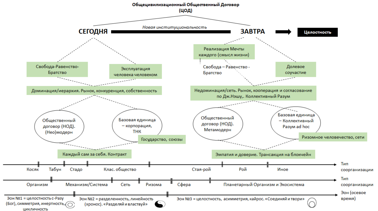
Рис. 1. Смена ЦОД
